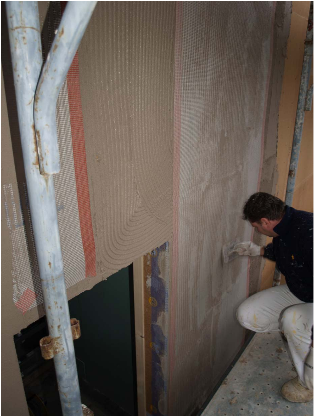
Inserimento della rete in fibra di vetro nella rasatura sul pannello in fibra di legno
