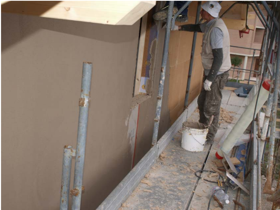
Posa della prima rasatura con rete sul cappotto in fibra di legno
