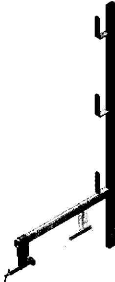
Fig. 9.1.2.1.1-1 Parapetto provvisorio ammorsato con ganascia fissa
